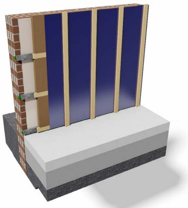
Houtvezel isolatie
