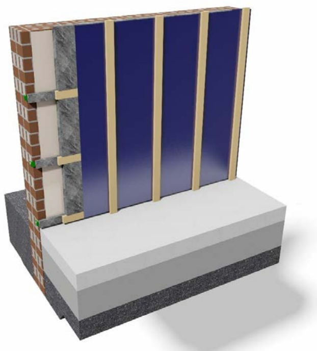
Aerogel isolatie
